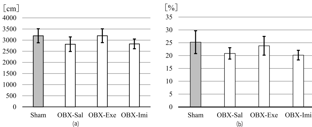
Fig. 5 : Y-maze test
